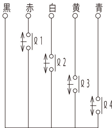
結線図
