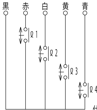
結線図
